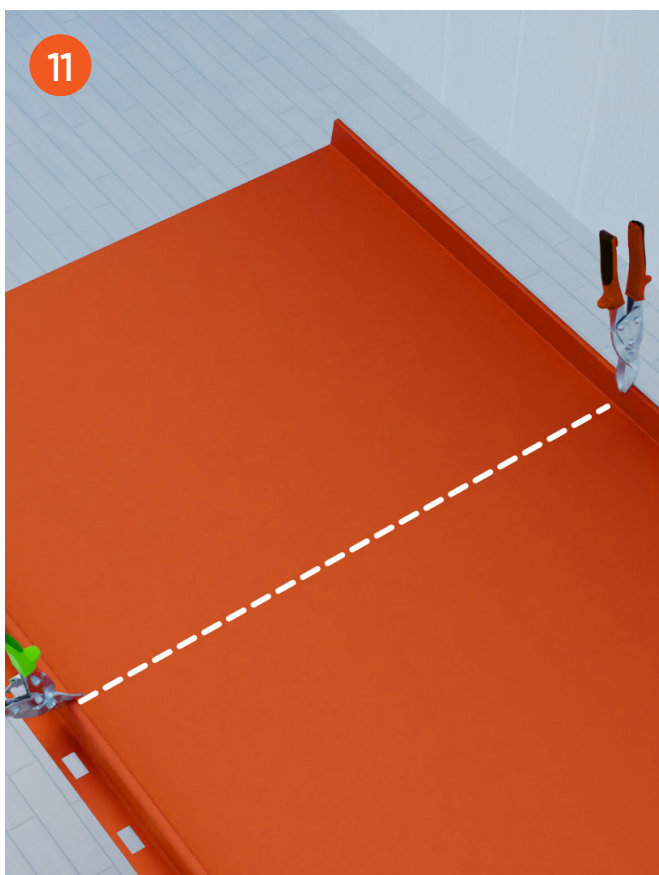
Klipp upp falsarna med hjälp av vänster och höger plåtsax.
