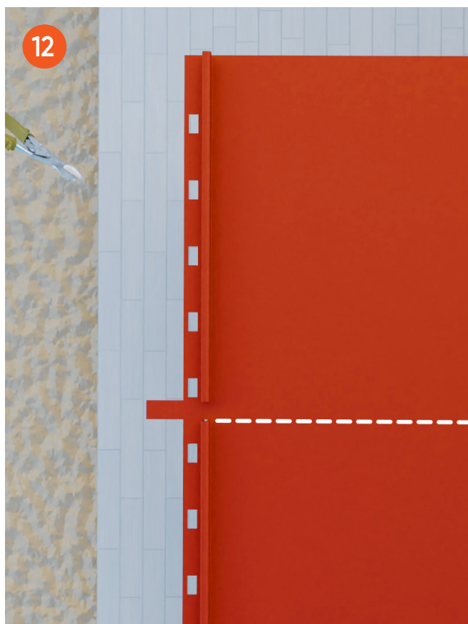
Vik ner urklippen på båda sidorna för att komma åt att kapa plåten.
